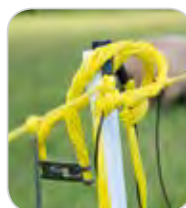
Edelstahlklemmen zur sicheren Verbindung von Netz zu Netz
