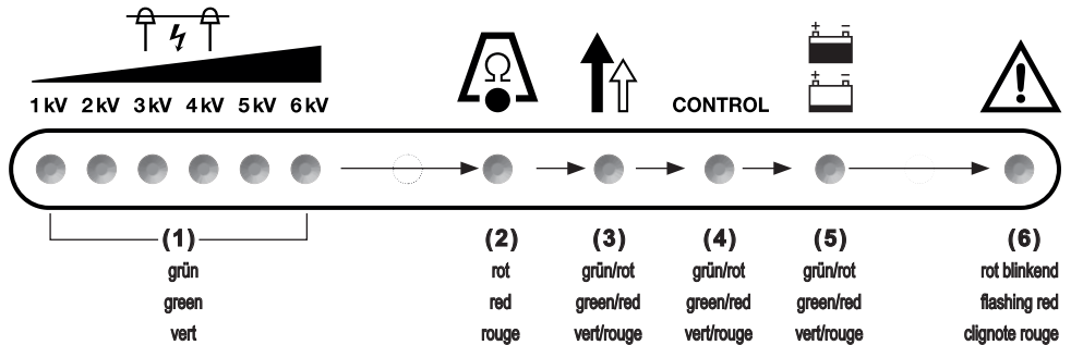
Fig. 3 / LED-Test
