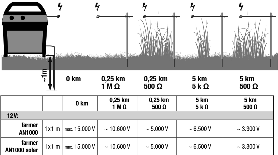
Fig. 8 CEE: de: max. Zaunlänge | en: max. fence line length | fr: longueur électrifiée pt: máximo comprimento de cerca | it: lunghezza massima recinto da: max. stängsellängd | nl: maximale afrasteringslengte | sk: maximálna dĺžka ohrady es: longitud máxima del vallado
