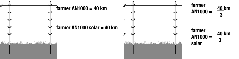
Fig. 8 CEE: de: max. Zaunlänge | en: max. fence line length | fr: longueur électrifiée pt: máximo comprimento de cerca | it: lunghezza massima recinto da: max. stängsellängd | nl: maximale afrasteringslengte | sk: maximálna dĺžka ohrady es: longitud máxima del vallado
