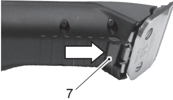
Fig. 6 Leikkuupään lukitus (7)
